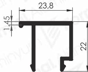
Pr.No: 9768 0,249 kg/m
