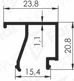
Pr.No: 4231 0,214 Kg/m
