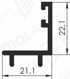
Pr.No: 9472 0,238 kg/m
