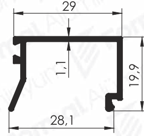
Pr.No: 9662 0,228 kg/m
