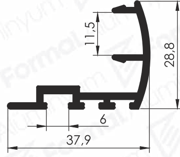
Pr.No: 2419 0,391 kg/m
