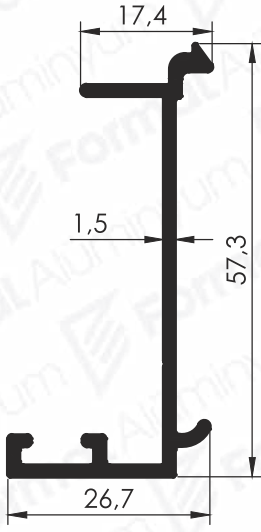
Pr.No: 9473 0,449 kg/m
