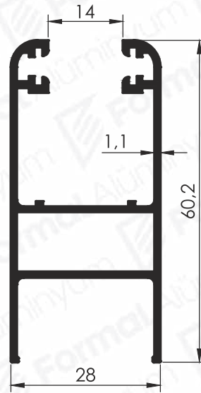
Pr.No: 2421 0,624 kg/m
