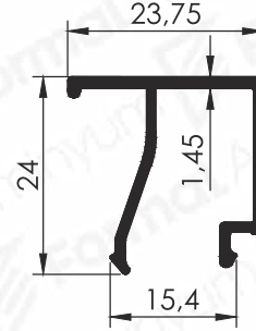
Pr.No: 3896 0,262 kg/m
