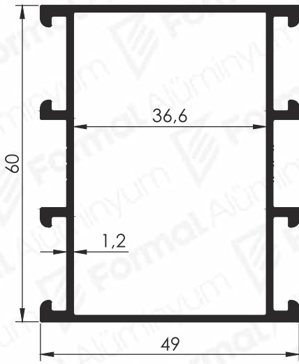
Pr.No: 4230 0,899 Kg/m
