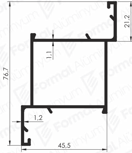
Pr.No: 2416 0,716 kg/m
