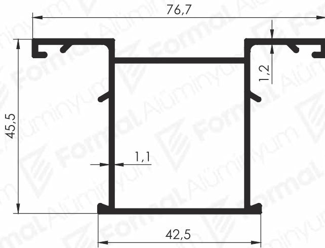
Pr.No: 2413 0,716 kg/m
