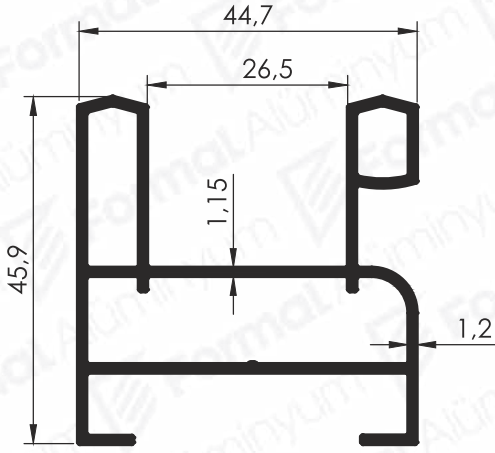
Pr.No: 2537 0,757 kg/m
