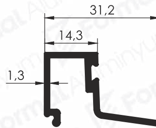
Pr.No: 2417 0,272 kg/m
