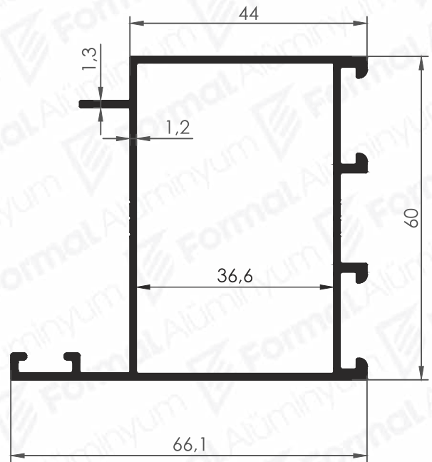
Pr.No: 4229 0,911 Kg/m
