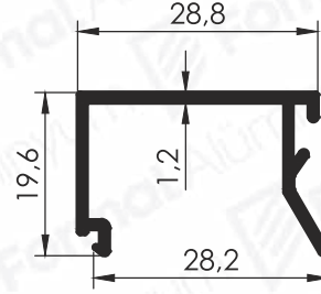
Pr.No: 2420 0,229 kg/m
