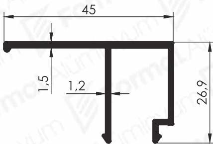
Pr.No: 9715 0,365 kg/m
