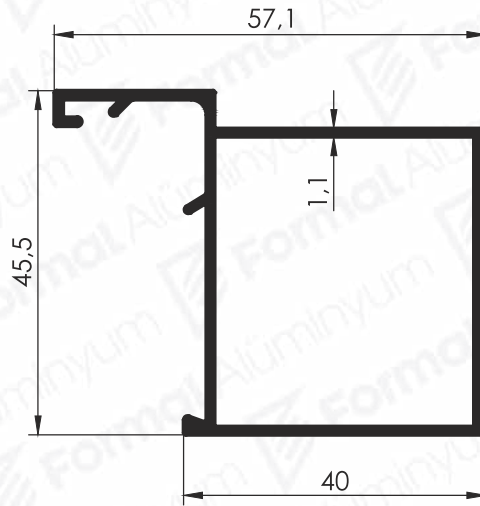
Pr.No: 2415 0,593 kg/m
