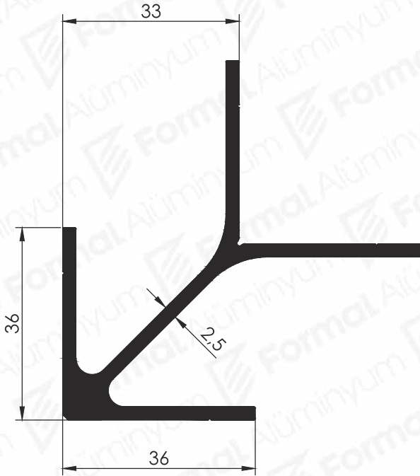
Pr.No: 9659 1,302 kg/m
