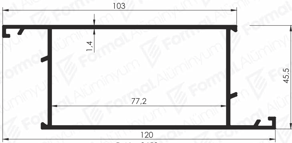
Pr.No: 9652 1,190 kg/m
