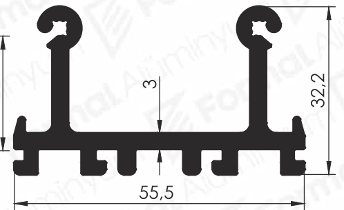
Pr.No: 9475 1,219 kg/m
