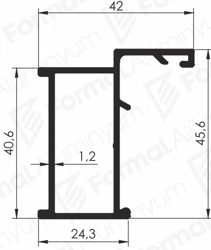
Pr.No: 2541 0,554 kg/m
