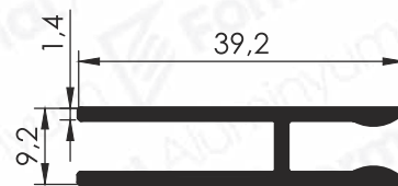
Pr.No: 8606 0,331 kg/m
