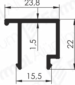
Pr.No: 9467 0,248 kg/m
