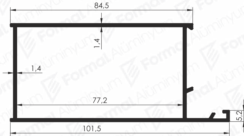
Pr.No: 1491 1,072 kg/m
