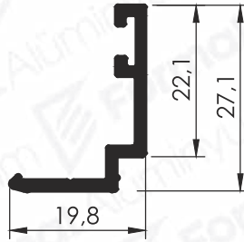
Pr.No: 1103 0,219 kg/m
