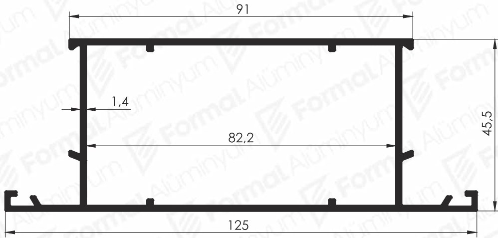
Pr.No: 9651 1,257 kg/m
