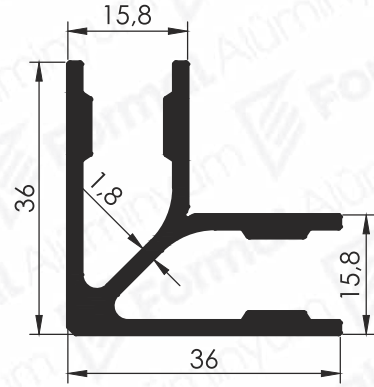
Pr.No: 9660 0,774 kg/m
