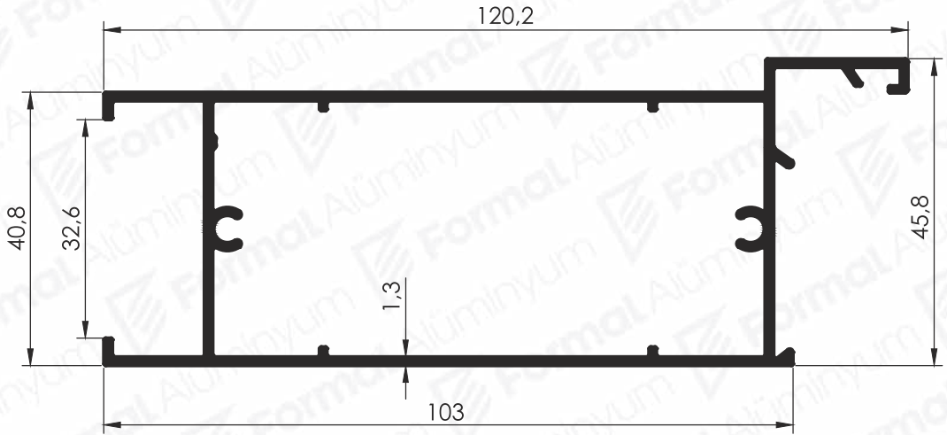
Pr.No: 2540 1,220 kg/m
