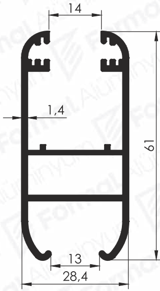
Pr.No: 2414 0,770 kg/m
