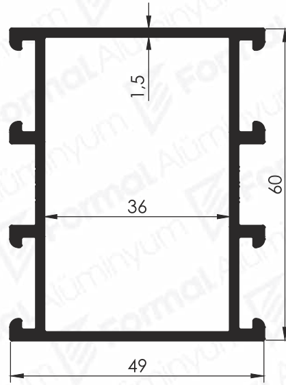
Pr.No: 9469 1,075 Kg/m
